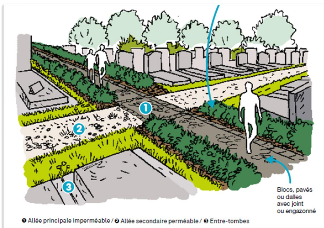
Figure 47 : Schéma d'aménagement d'un cimetière écologique (FLANDIN, 2022)
